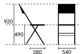
Dimensions en millimètre Measurements in millimeter
