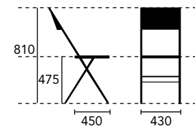
Dimensions en millimètre Measurements in millimeter
